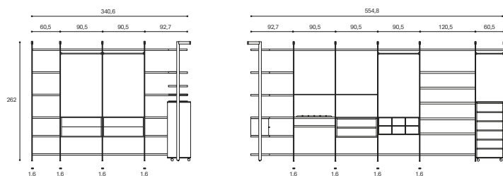
Cabina montanti L.340,6x554,8 H.262 P.41 cm
